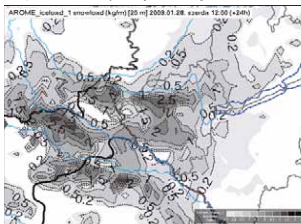
10. ábra: Várható akumulált hőteher az AROME 12 UTC-s futtatásának 24. órájában (január 28. 12 UTC). A maximális értékek 2,5 kg/m körül adódnak.
