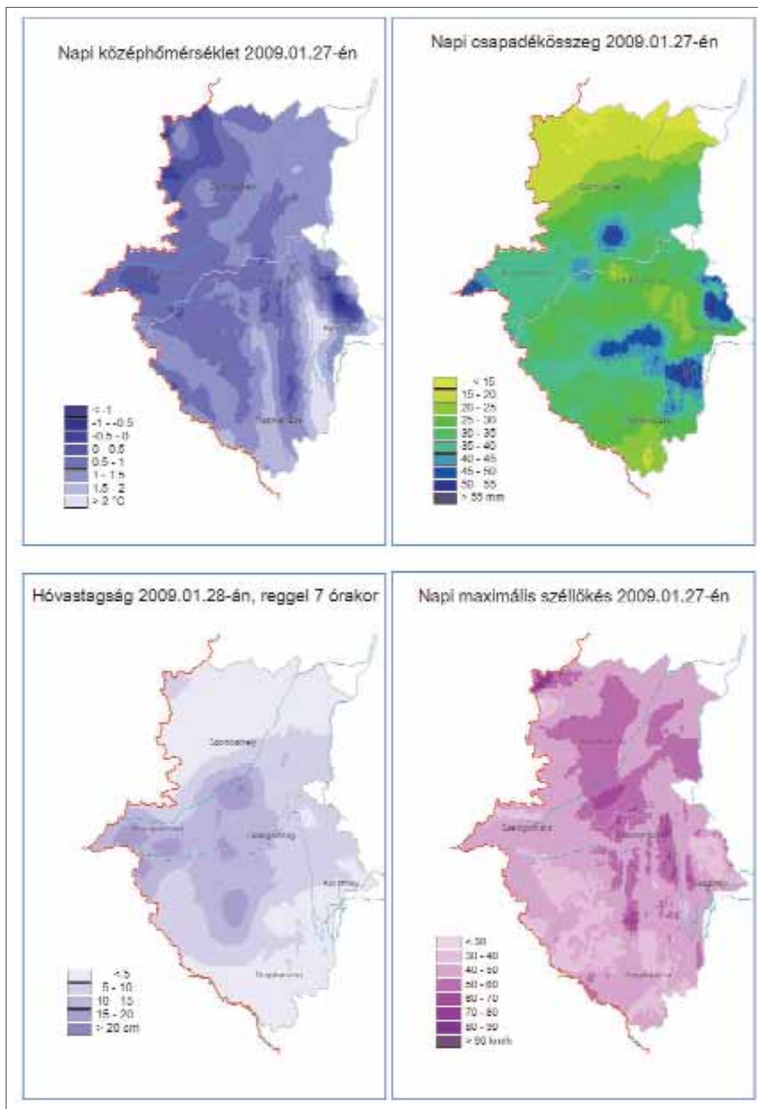
1. ábra Néhány meteorológiai paraméter térbeli eloszlása 2009.01.27-én Vas és Zala megye területén
