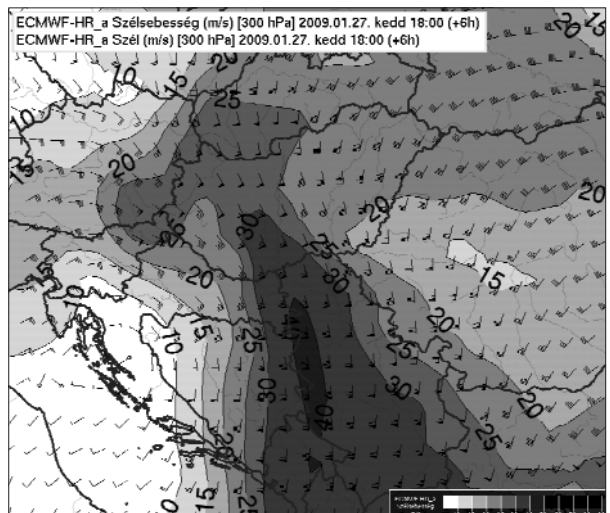
5. ábra: 300 hPa-os áramlás (január 27. 18 UTC). A Dunántúl nyugati része a mediterrán ciklon frontrendszerének okklúziós pontja közelében és egyben a futóáramlás bal-kilépő zónája alatt helyezkedik el. A futóáramlás magjában hazánkhoz közel a 40 m/s-os izotachák is megjelennek.
