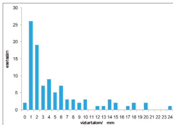
4. ábra A Szentgotthárdon megfigyelt tapadó havas lerakódások vízartalmának histogramja
