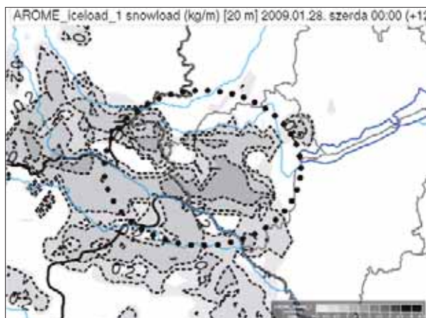
9. ábra: Várható akumulált hőteher az AROME 12 UTC-s futtatásának 12. órájában (január 28. 00 UTC). A maximális értékek 1 kg/m körül adódnak. A tapadó hóhoz köthető 27-i esti káresemények helyszínei hozzávetőlegesen a pontozott ellipszisen belülre esnek.
