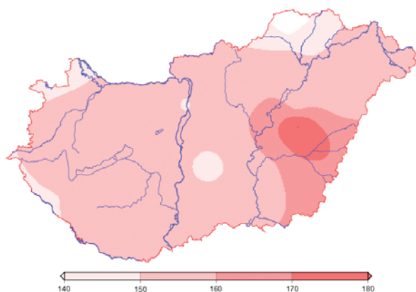
3.ábra: A tavasz globálisugrás összege MJ/cm²-ben
