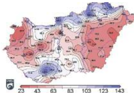
9. ábra. A 2010. május 30. 06 UTC és június 5. 06 UTC között lehullott csapadék összege
