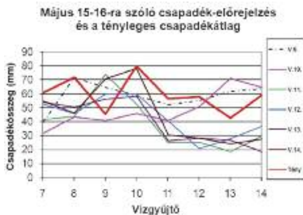
20. ábra. A 2010. május 15–16-ra szóló csapadék-előrejelzés és a tényleges csapadékátlag Vízgyűjtők: 7 – Vág, Garam, Ipoly; 8 – Közép-Dunavölgy; 9 – Zala, Balaton; 10 – Kapos, Sió; 11 – Sajó, Hernád; 12 – Zagyva; 13 – Közép-Tiszavölgy; 14 – Bodrog
