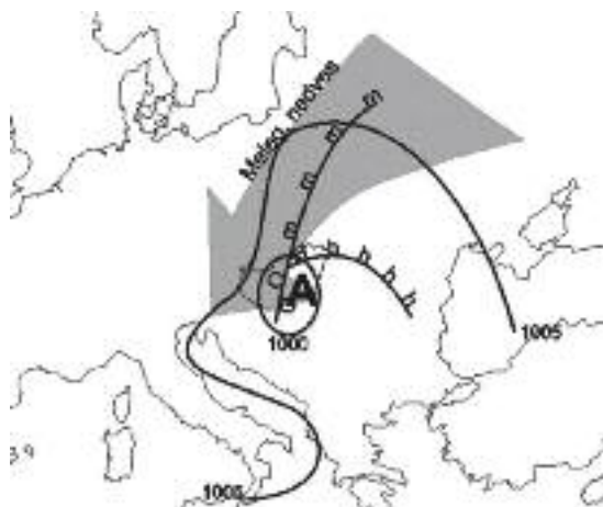
11. ábra. A 2010. június 1. 12 UTC-s időjárási helyzet sematikus képe a meleg, nedves szállítószalaggal
