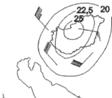
8. ábra. A potenciálisan kihullható vízmennyiség eloszlása a Kárpát-medencében 2010. május 16. 00 UTC-kor
