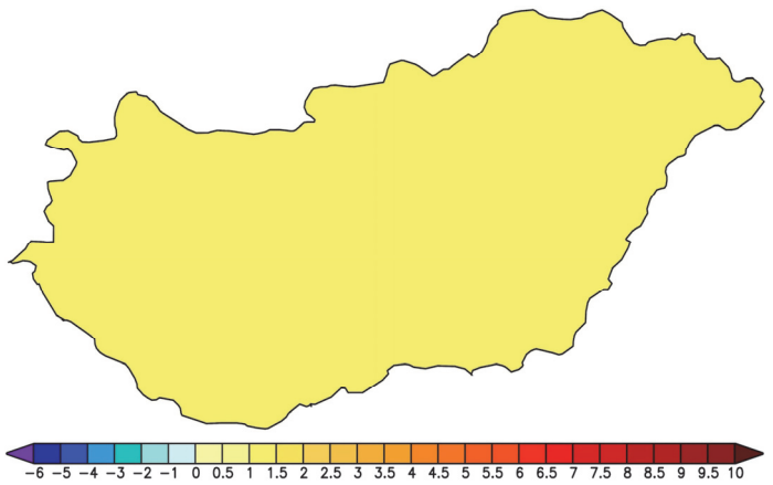
20. ábra: A REMO modell előrejelzése évi előrejelzés a 2021-2050-es időszakra (Bartholy et al. 2011b)
